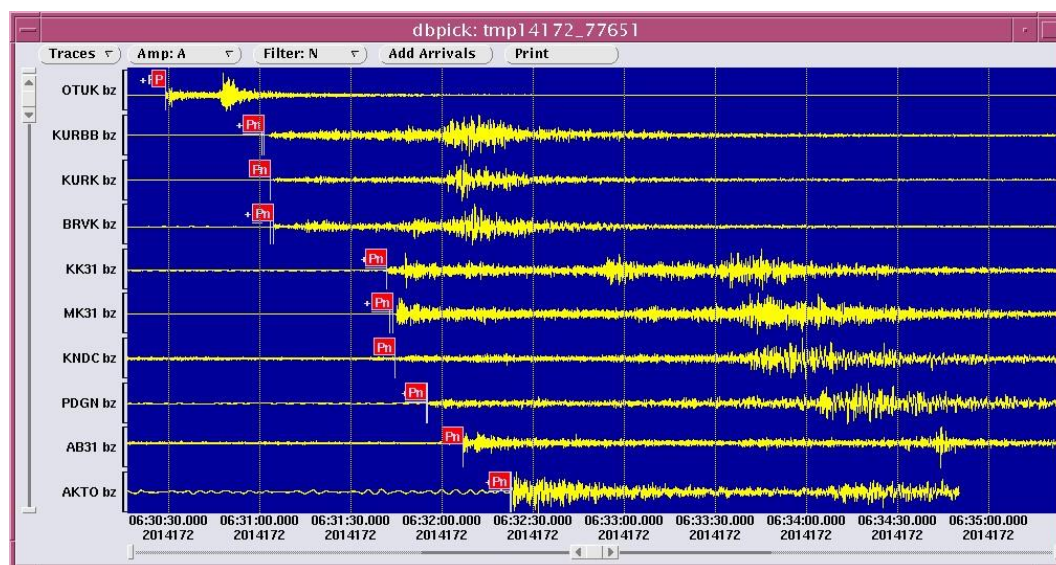
Рисунок 4. Записи Карагандинского землетрясения на станциях ИГИ (вертикальные компоненты)
