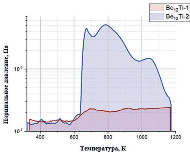
Рисунок 4. Спектры газовыделения по сигналу \text{D}_2 из образцов БТ-1 и БТ-2
