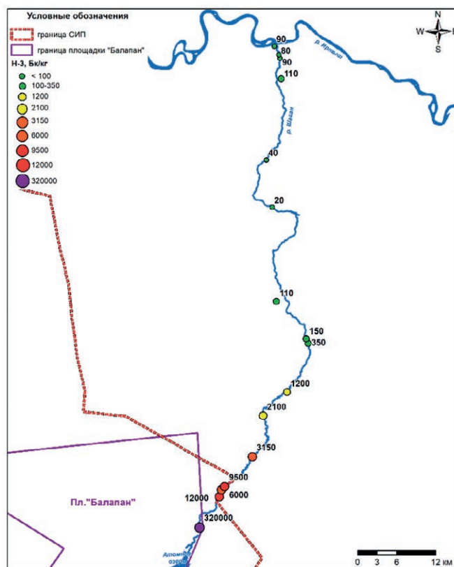
Рисунок 3. Результаты определения содержания ^3\text{H} в воде реки Шаган [18]
