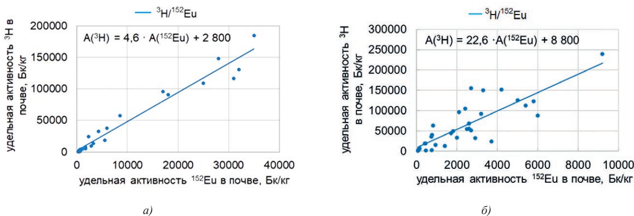
Рисунок 1. Зависимость удельной активности ^3\text{H} от удельной активности ^{152}\text{Eu} в почве: а - площадка «Опытное поле», техническая площадка П-1; б - территория «Атомного» озера [5]
