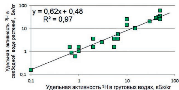
Рисунок 2. Зависимость содержания ^3\text{H} в свободной воде растений-фреатофитов от содержания ^3\text{H} в грунтовых водах [10]
