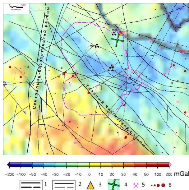
1 – основные разломы в коренных породах (сплошная линия) и перекрытые рыхлыми отложениями (пунктир); 2 – второстепенные разломы; 3 и 4 – сейсмические станции Курчатов и Курчатов-Крест, соответственно; 5 – карьер; 6 – эпицентры землетрясений по возрастанию энергетического класса для значений <5; 9; 12,5; ≥15;
