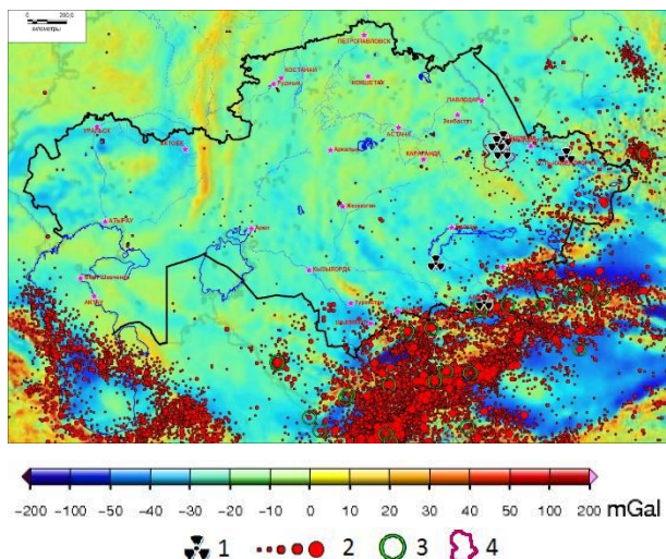
1 – объекты атомной отрасли в Казахстане; 2 – эпицентры землетрясений по возрастанию энергетического класса для значений <5; 9; 12,5; ≥15; 3 – эпицентры катастрофических землетрясений; 4 – контур СИП
