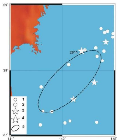
Эпицентры землетрясений: 1 – M=5,9 ; 2 – M=6,0-6,9 ; 3 – M=7,0-7,9 ; 4 – Mw=9,0 (указан год); 5 – кольцевая структура
