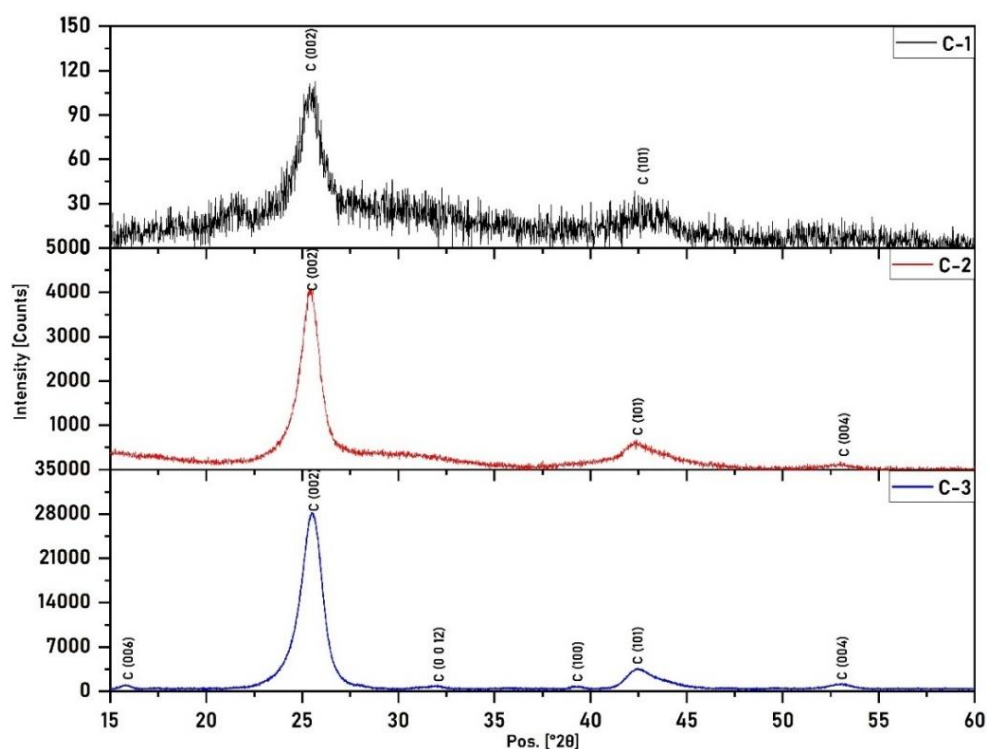
3-сурет – C-1, C-2, C-3 үлгілерінің 15–60° 2θ бұрыштық диапазонында алынған дифрактограммаларының қабаттаса салынған көрінісі
